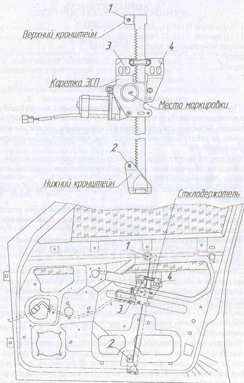
Установка ЭСП в переднюю правую дверь. Рис. 1.
