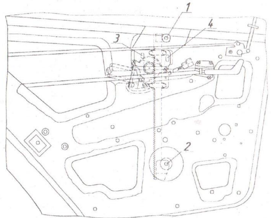
Установка ЭСП VA3 2110/2170 (Приора) в заднюю левую дверь. Рис. 2.
