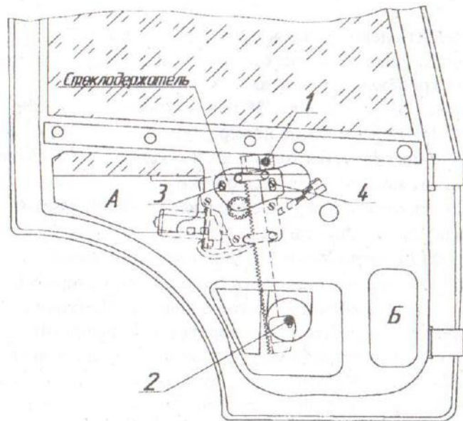
Установка ЭСП VA3 2123 Niva Chevrolet в заднюю левую дверь. Рис. 1.
