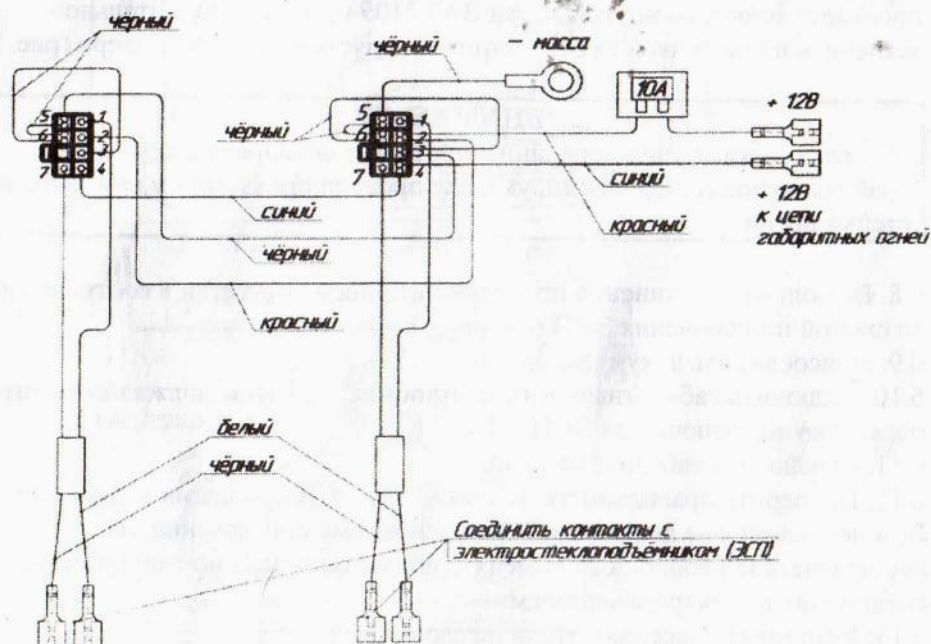
Рис. 4. Схема подключения электростеклоподъёмников к бортовой сети автомобиля.
