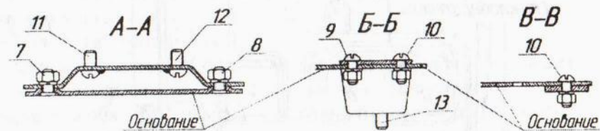
Крепление кронштейнов к основанию рис. 2.
