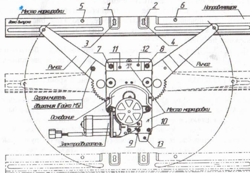
Электростеклоподъемник рис. 1
