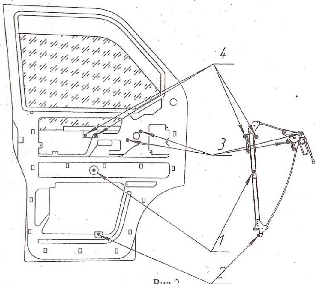
Рис.2 Установка ЭСП в левую дверь
